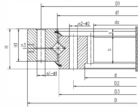
内齿 Internal Gear
